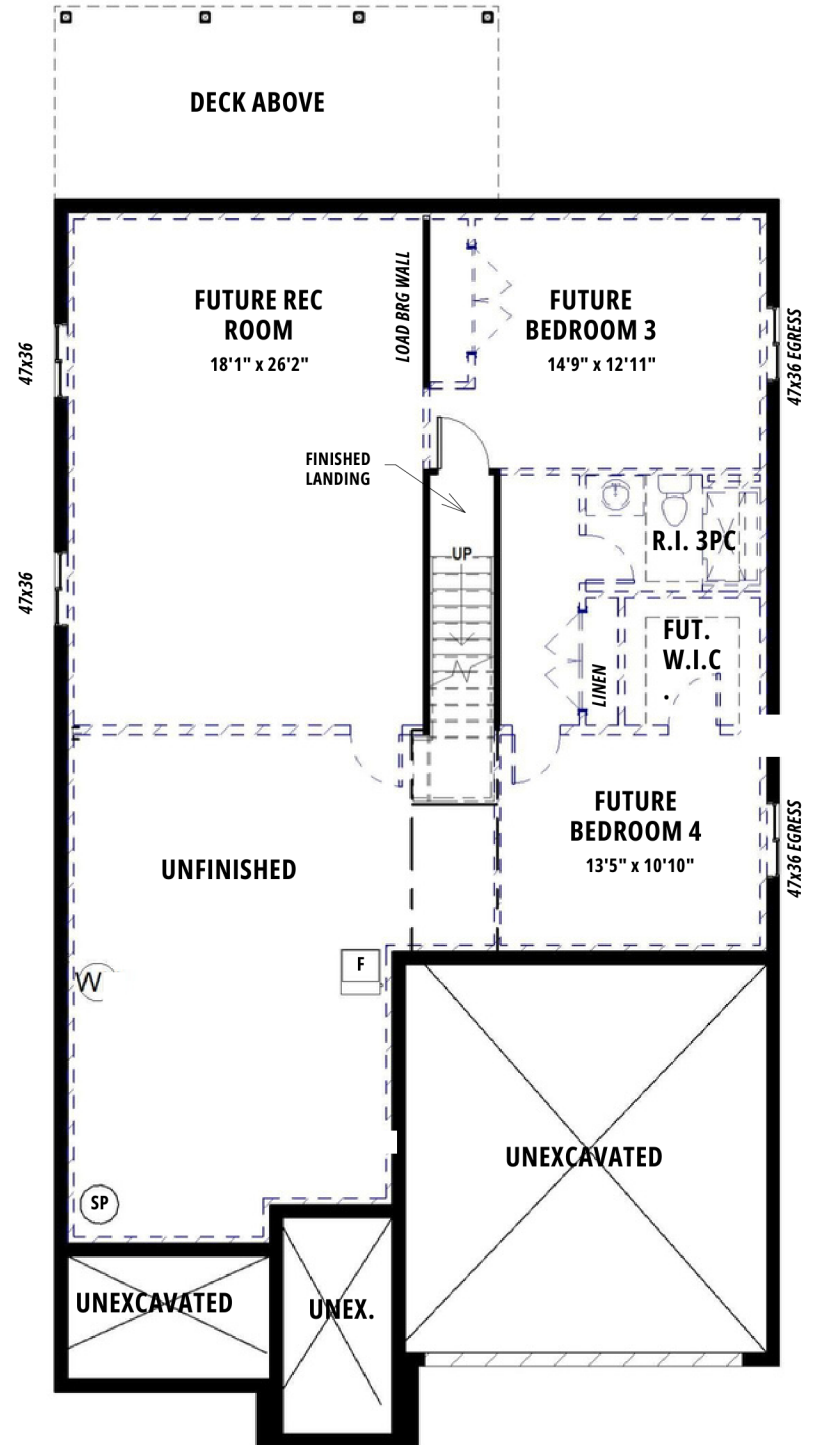
BASEMENT | 8'4" POUR
