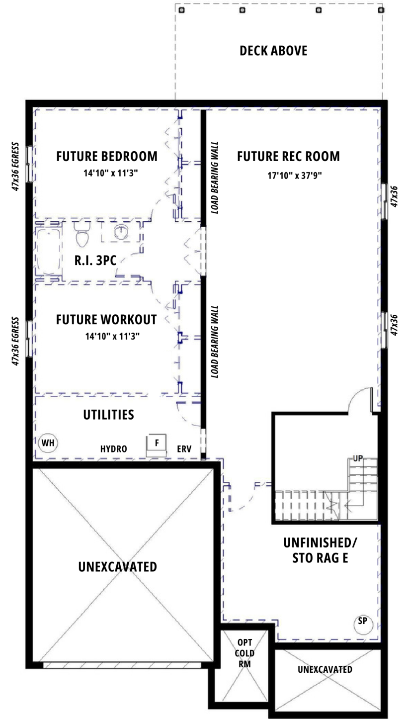
BASEMENT | 8'4" POUR
