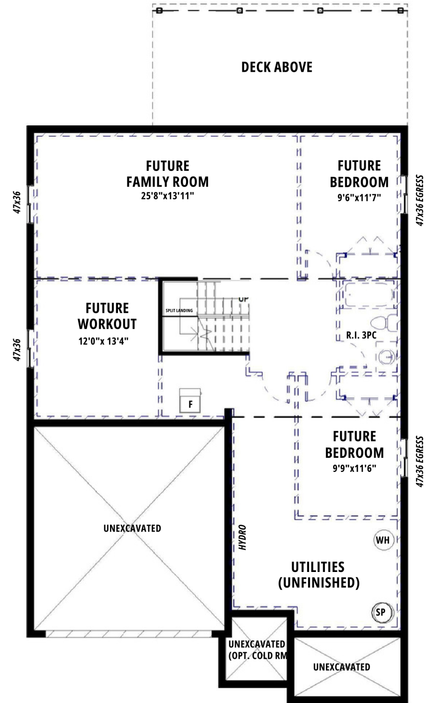
BASEMENT | 8'4" POUR
