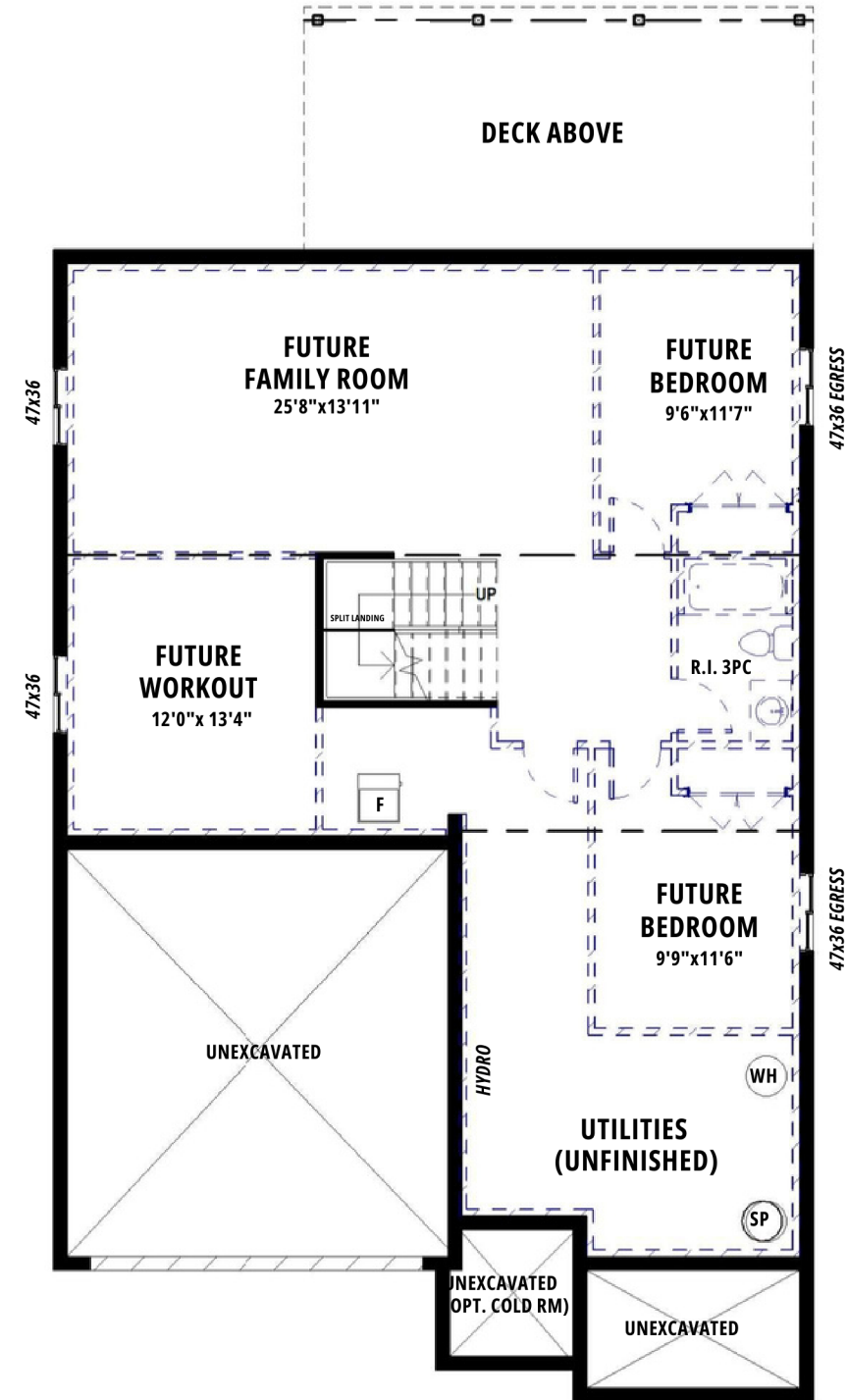
BASEMENT | 8'4" POUR
