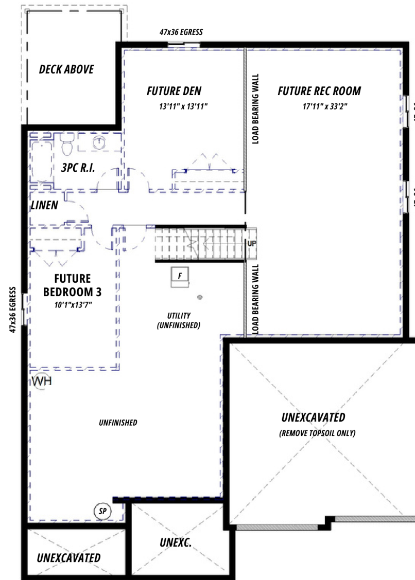
BASEMENT | 8'4" POUR
