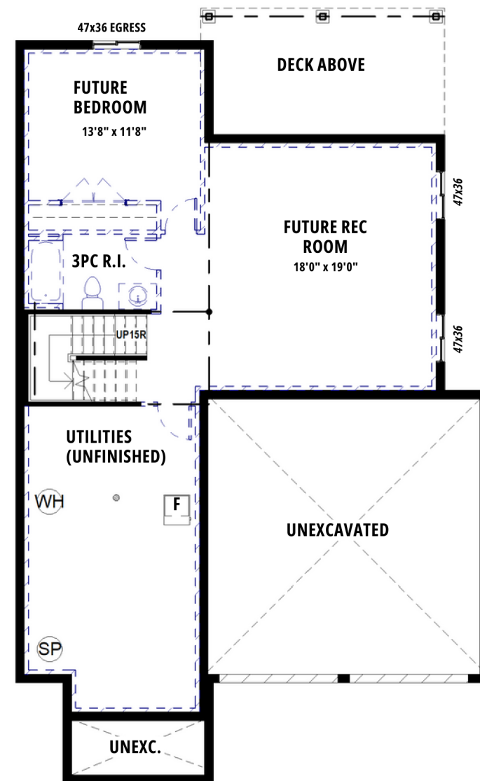
BASEMENT | 8'4" POUR
