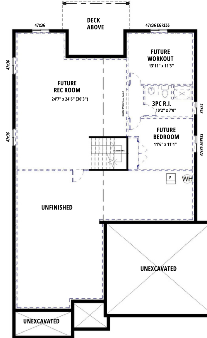
BASEMENT | 8'4" POUR
