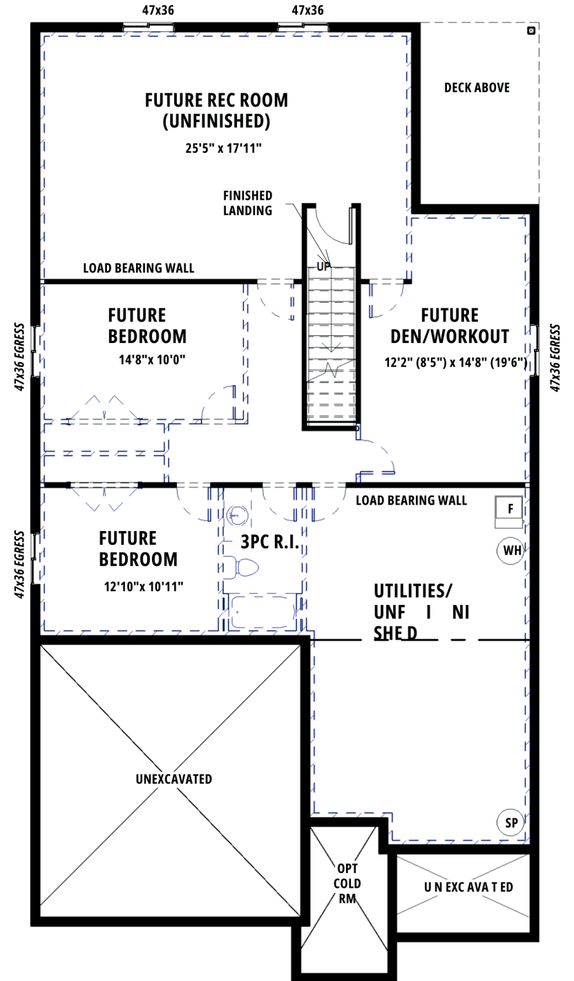
BASEMENT | 8'4" POUR
