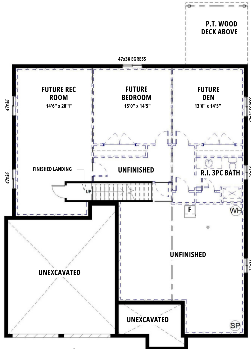
BASEMENT | 8'4" POUR
