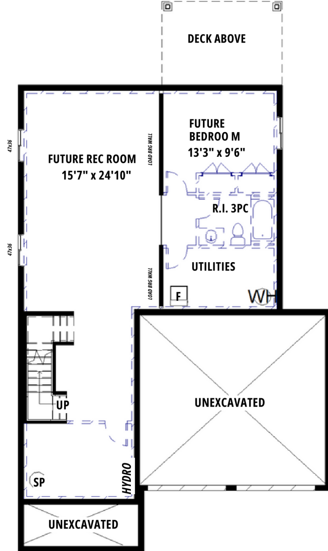
BASEMENT | 8'4" POUR
