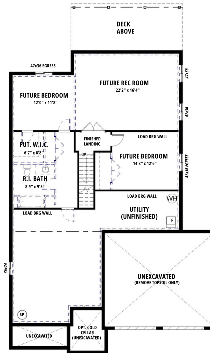
BASEMENT | 8'4" POUR
