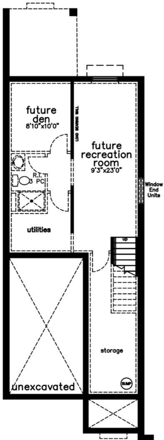
Basement - 7'10" Pour
