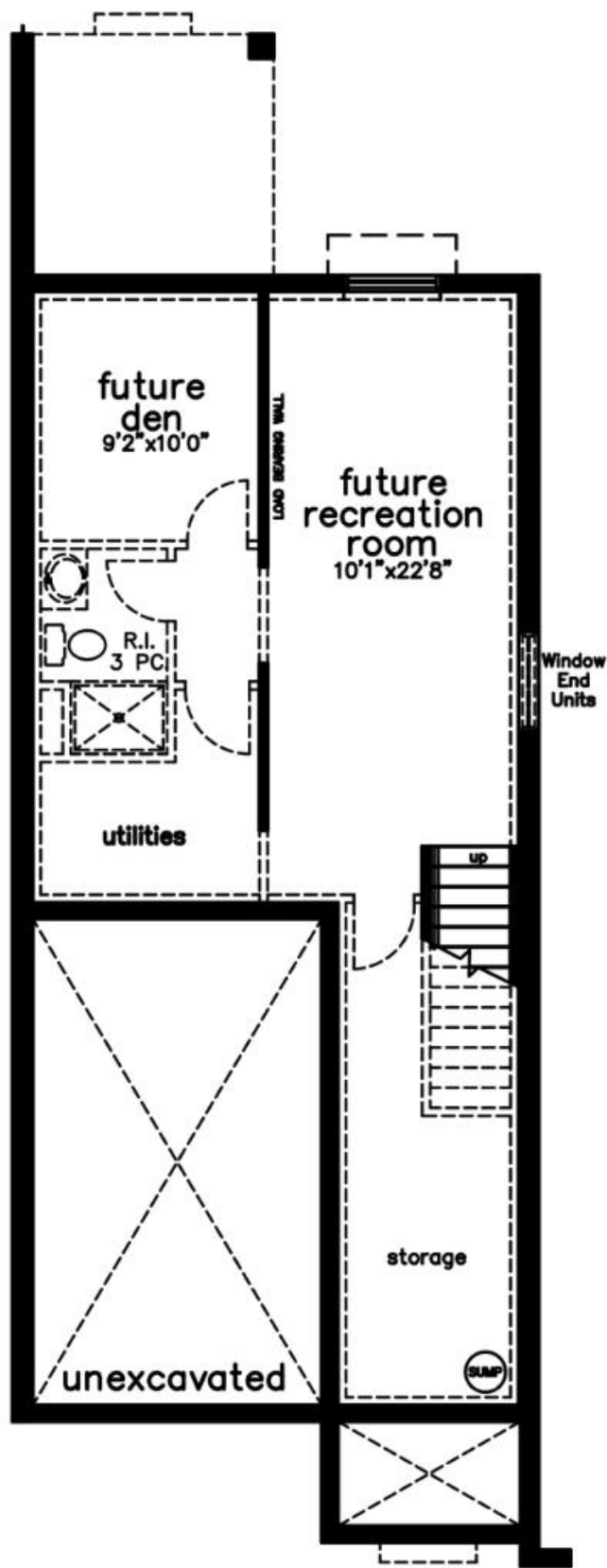
Basement - 7'10" Pour
