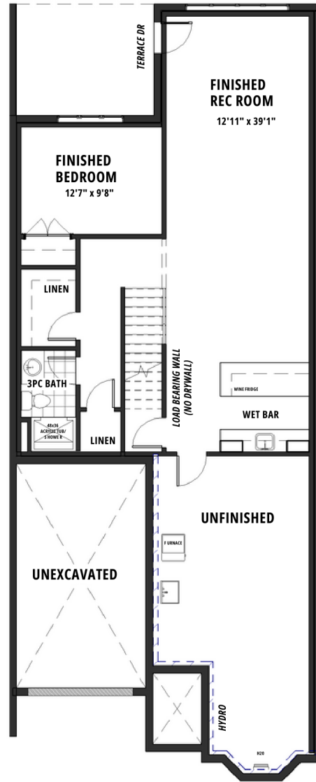
BASEMENT 1002 SQ FT [8'4" POUR]
