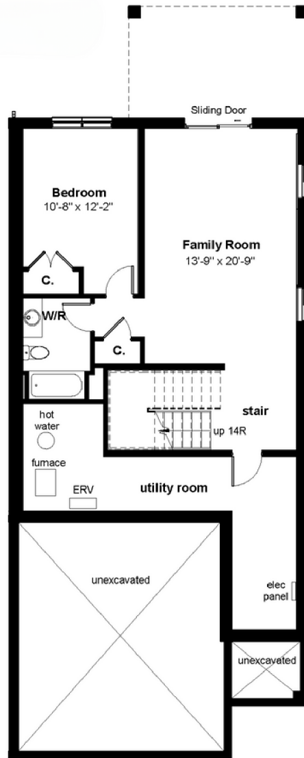
BASEMENT 654 SQ FT [8'4" POUR]
