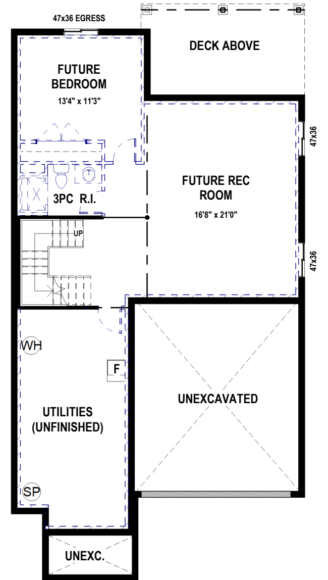
BASEMENT - 8'4" POUR
