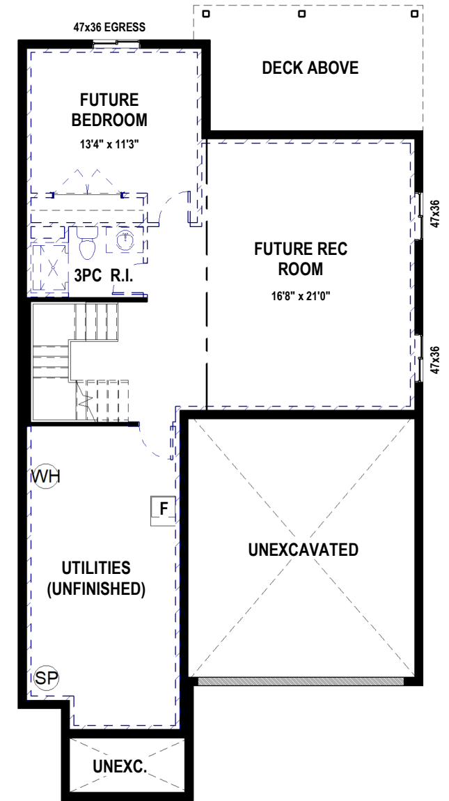
BASEMENT - 8'4" POUR
