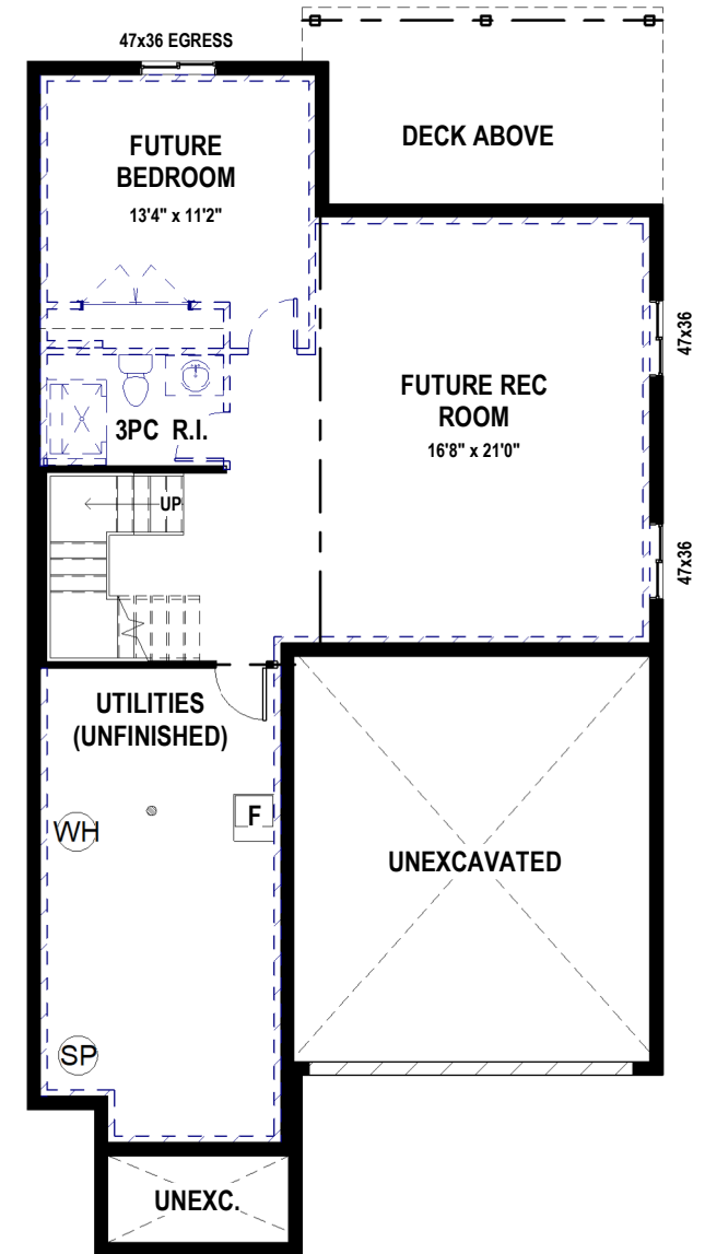
BASEMENT - 8'4" POUR
