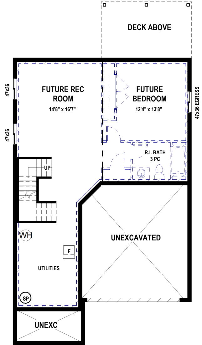
BASEMENT - 8'4" POUR
