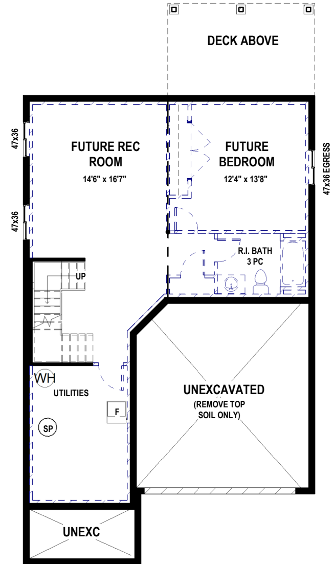
BASEMENT - 8'4" POUR
