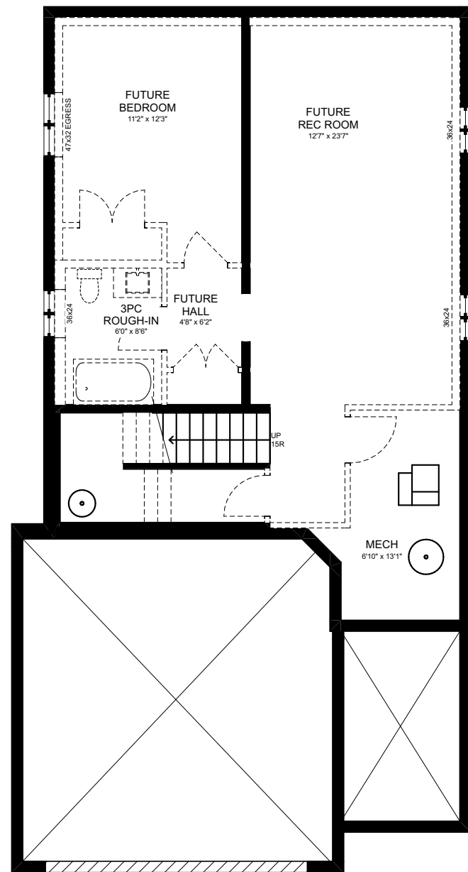
BASEMENT - 8'4" POUR
