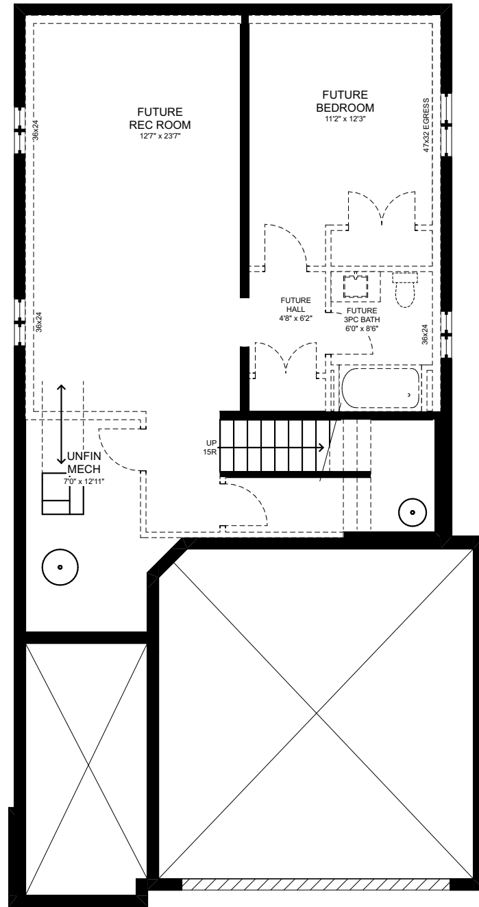
BASEMENT - 8'4" POUR
