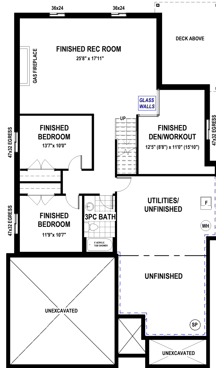
BASEMENT - 1212 SQ.FT. FINISHED AREA - 8'4" POUR
