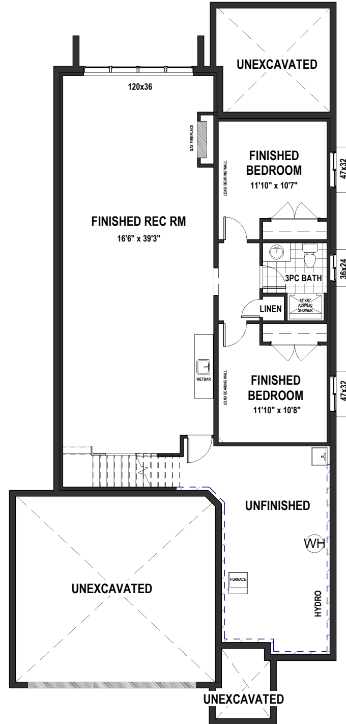
BASEMENT - 1203 SQ.FT. FINISHED AREA - 8'-4" POUR
