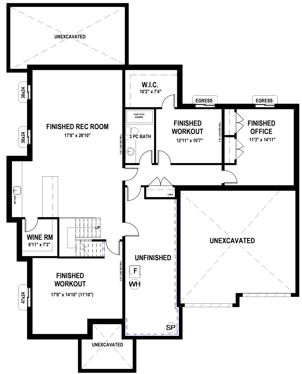
BASEMENT - 1613 SQ.FT. FINISHED AREA - 8'6" POUR
