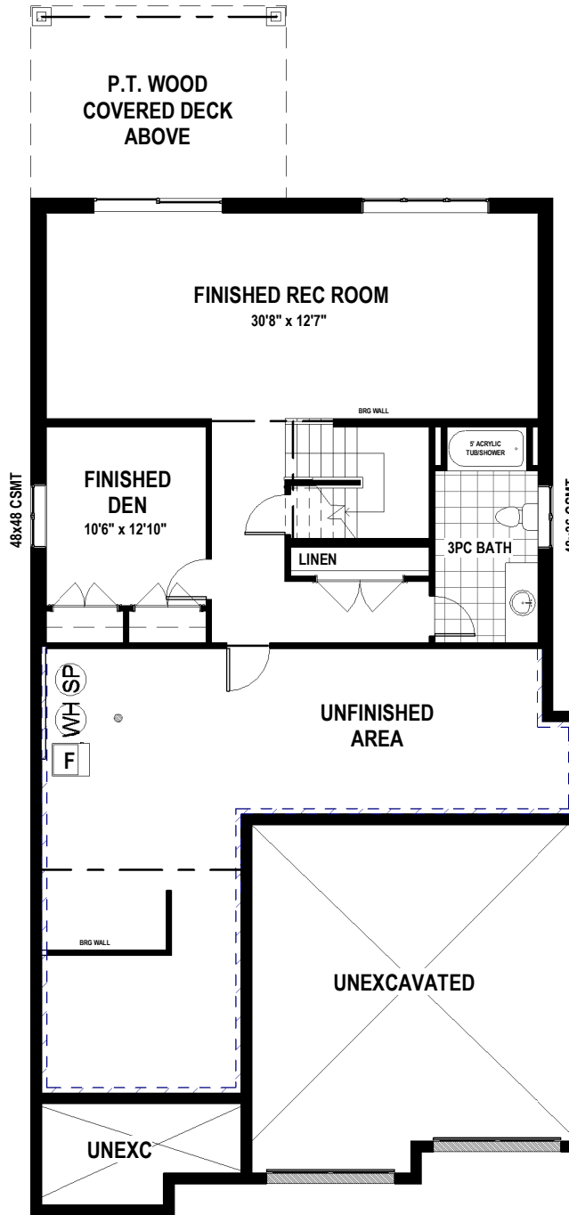
BASEMENT - 859 SQ.FT. FINISHED AREA - 7'10" POUR
